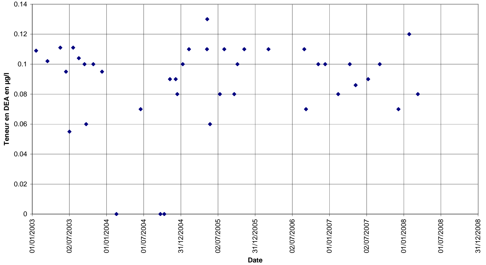
Forage F4 : évolution de la teneur en deséthylatrazine
