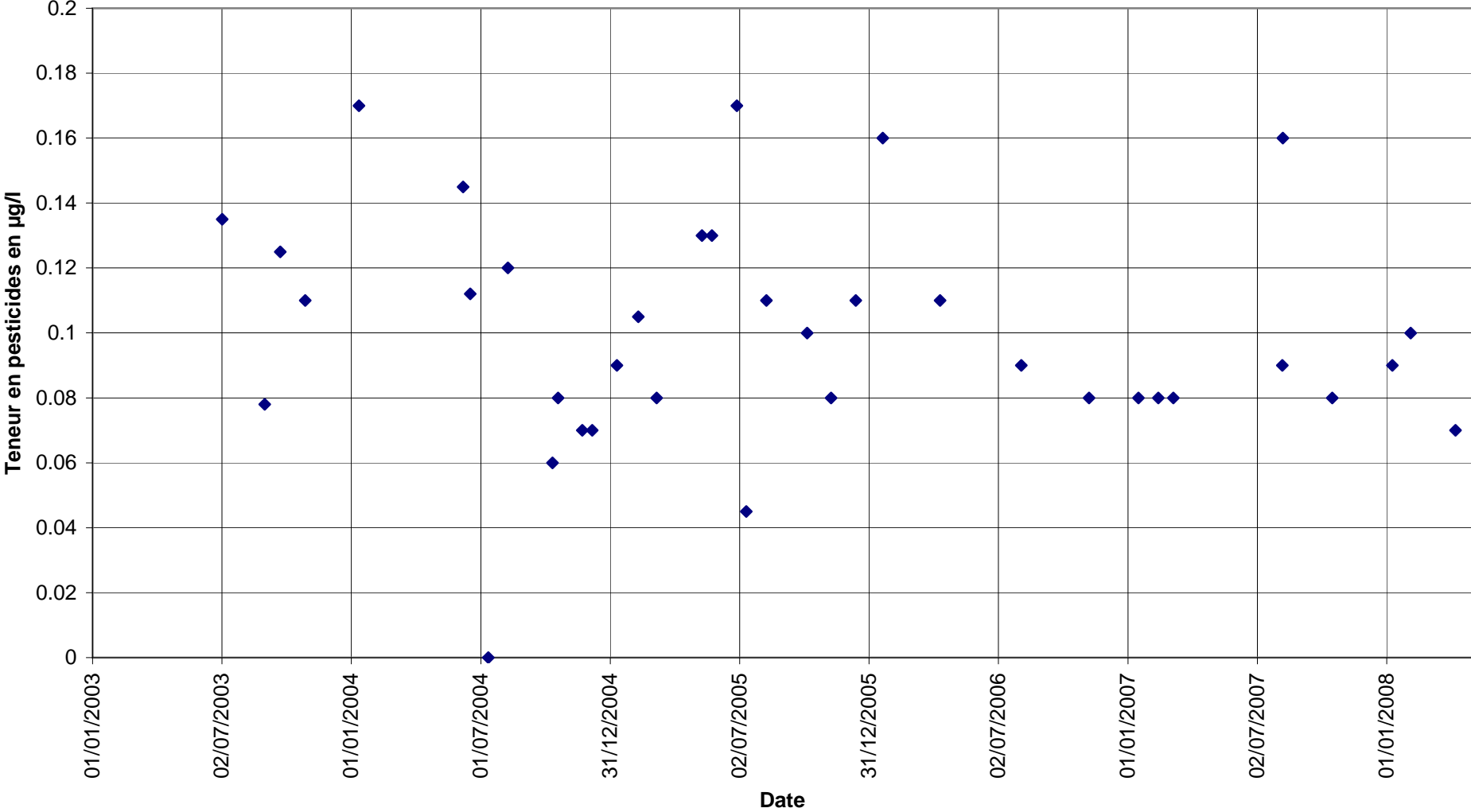
Forage F2 : évolution de la teneur en pesticides totaux
