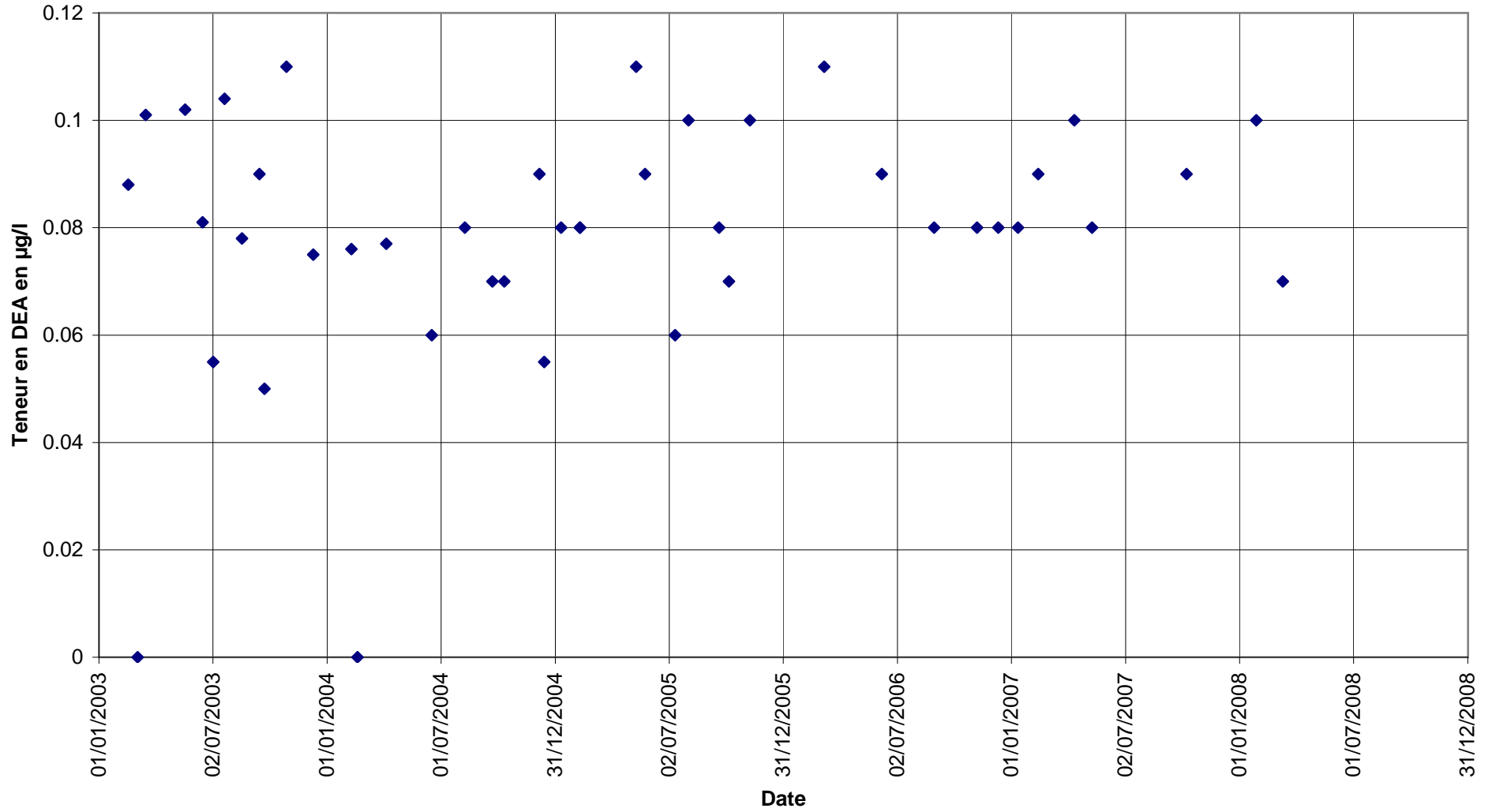
Forage F2 : évolution de la teneur en deséthylatrazine
