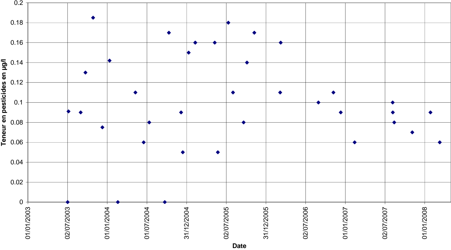
Forage F1 : évolution de la teneur en pesticides totaux
