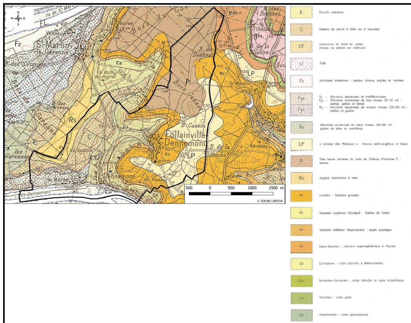
Illustration 1 : extrait de la carte géologique de Mantes-la-Jolie
