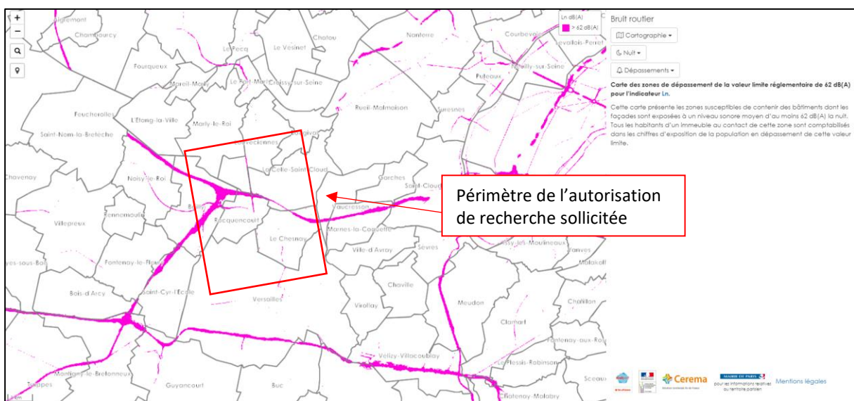
Figure 90 – Carte des zones de dépassement de la valeur réglementaire de 62 dB(A) pour l'indicateur Ln
