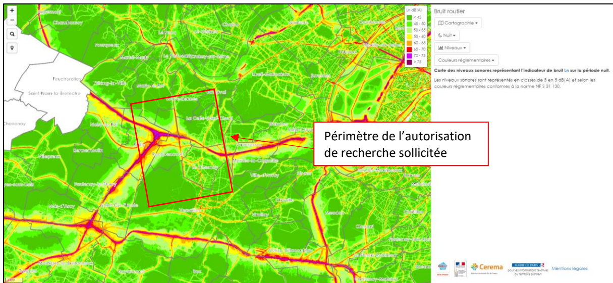
Figure 89 – Carte des niveaux sonores représentant l'indicateur Ln sur la période nuit
