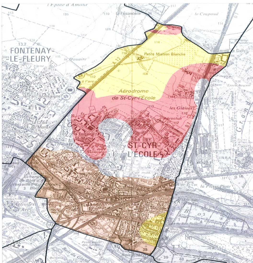
Illustration 4 : Carte d'aléa retrait-gonflement des argiles sur la commune de Saint-Cyr-l'Ecole
