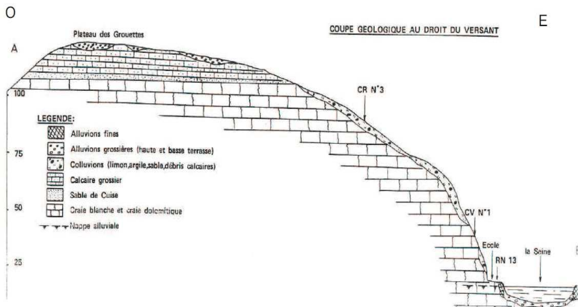
Illustration 2 : coupe géologique au droit de la commune de Rolleboise (source : LROP dossier 26111 en 1991-1992)
