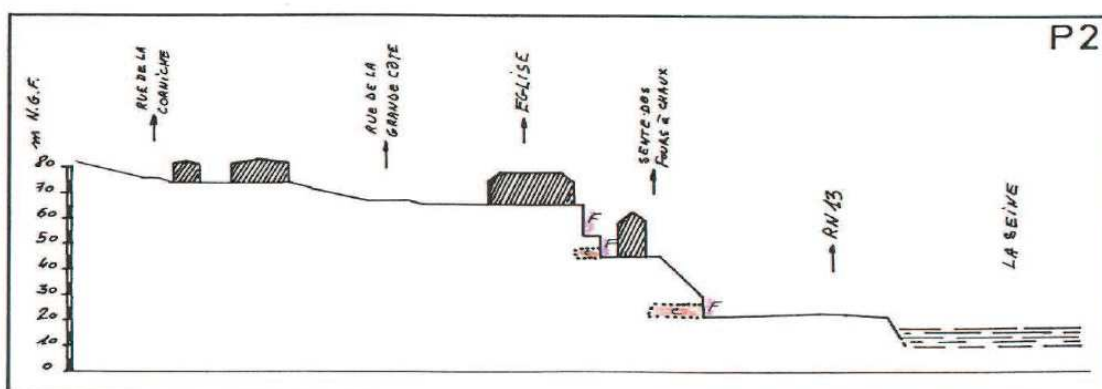
Illustration 1 : profil de versant (source : dossier LREP, dossier 2.4.13649 d'avril 1995)
